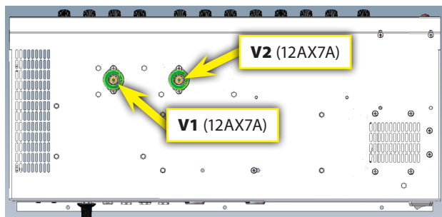
(Chassis, Unterseite)
