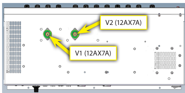
(Šasi zespodu)
